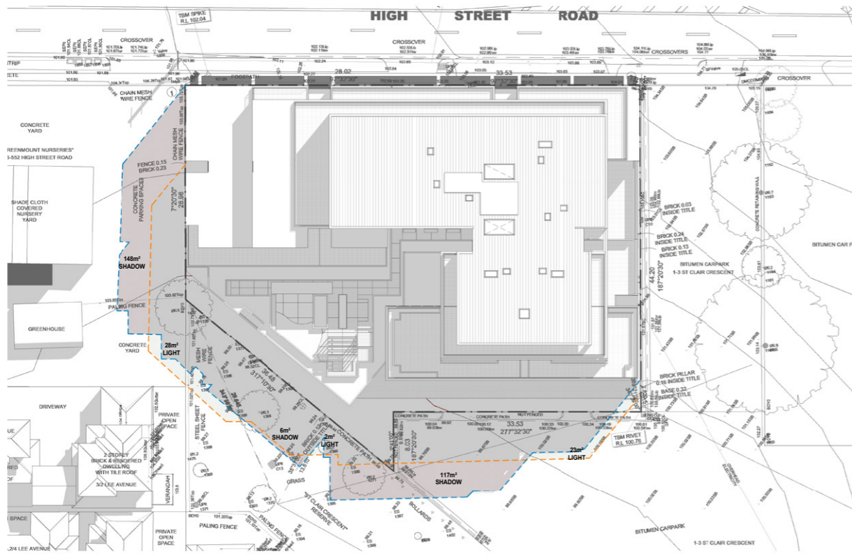
3 SHADOW 11AM 1 : 250
