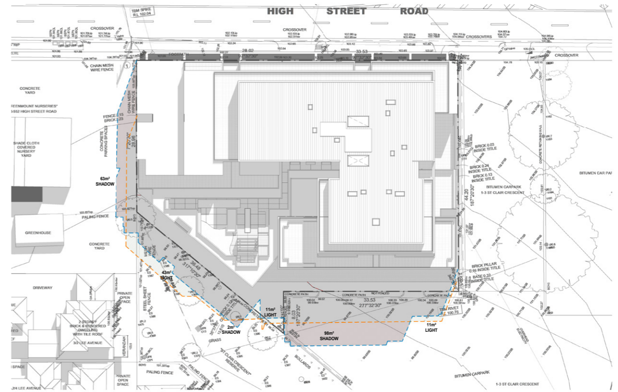
4 SHADOW 12PM 1 : 250
