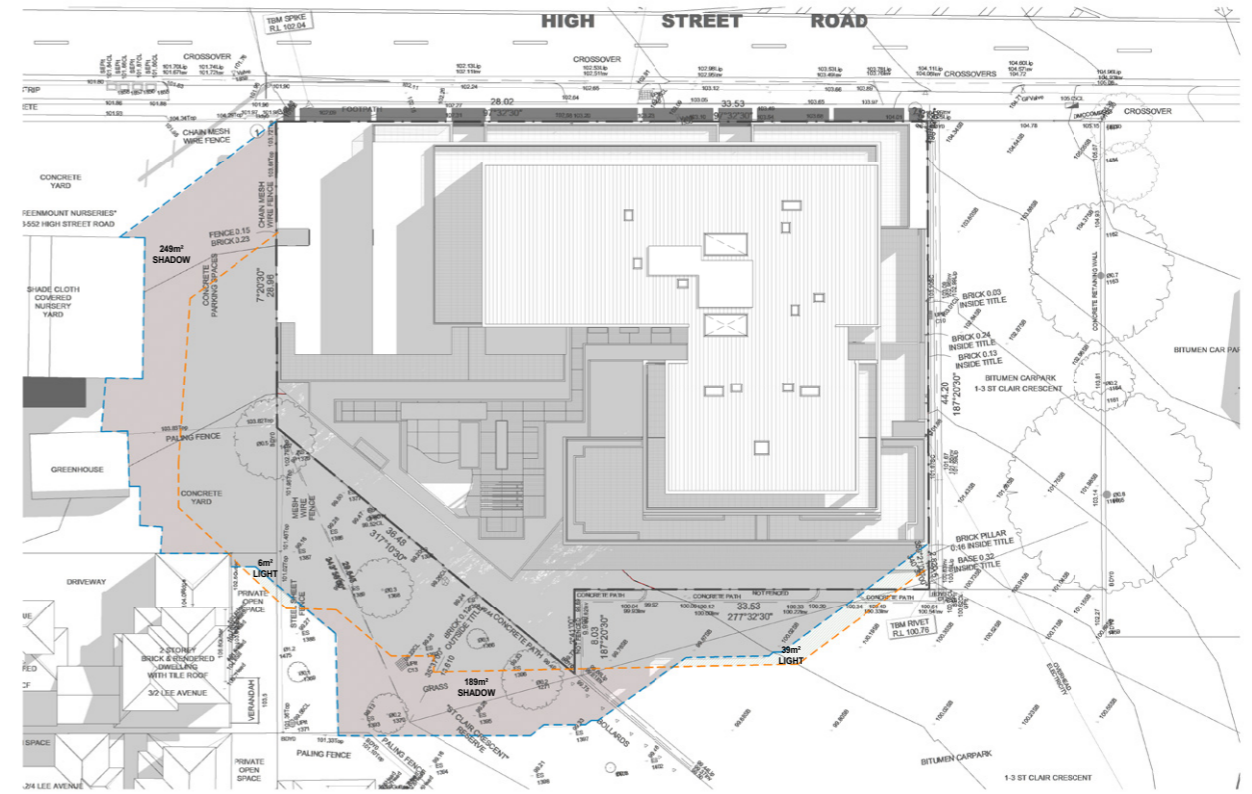
2 SHADOW 10AM 1 : 250
